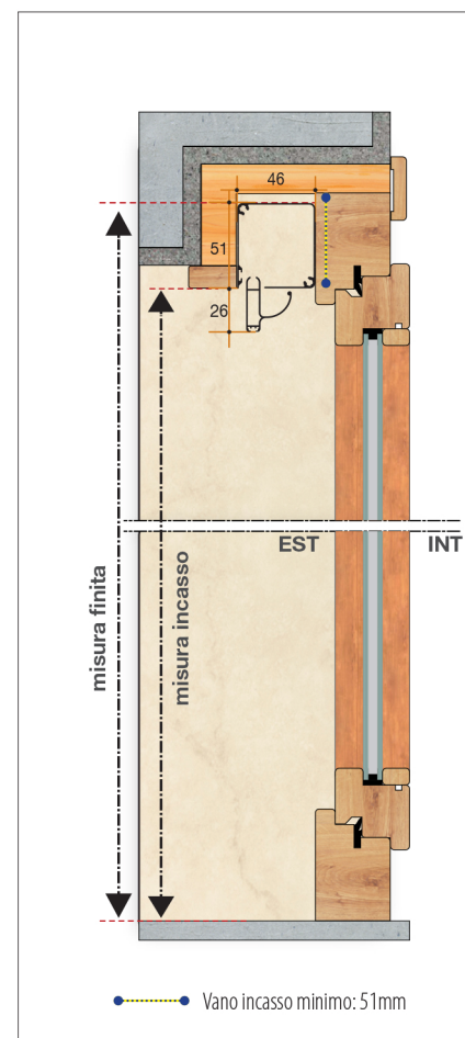
Sezione verticale
